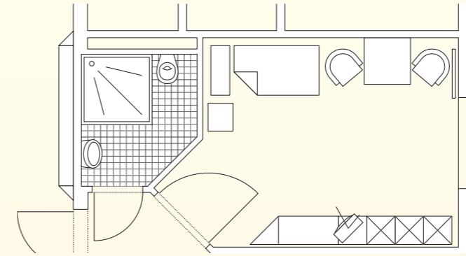
Beispiel-Grundriss eines unserer 122 Einzelzimmer.
